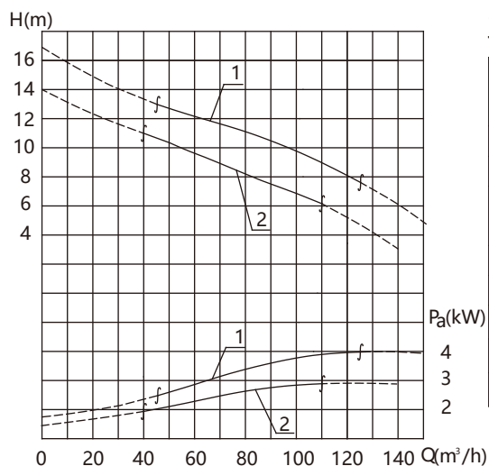
性能曲线图
