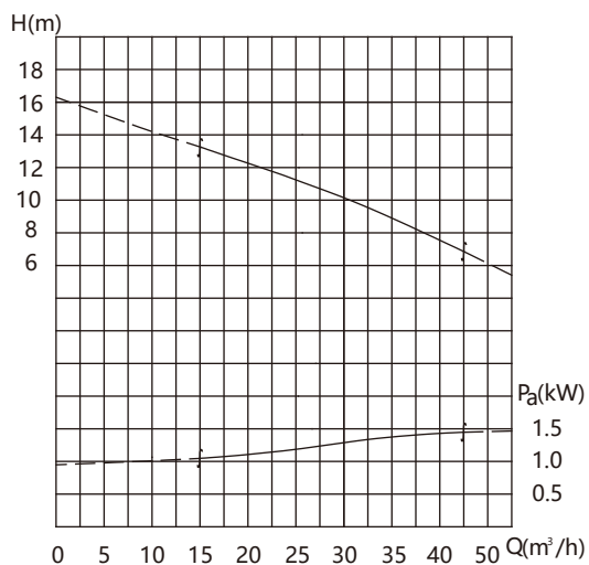
性能曲线图
