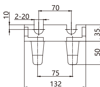
B 向
