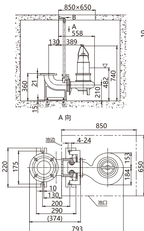
安装尺寸图
