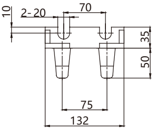
B 向
