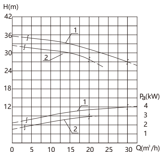
性能曲线图
