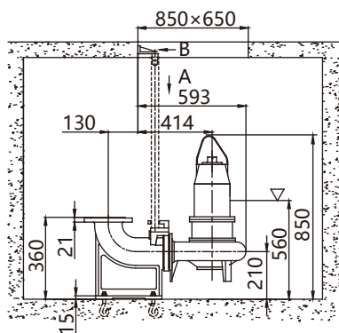
A 向
