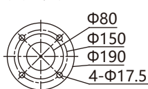
法兰尺寸
