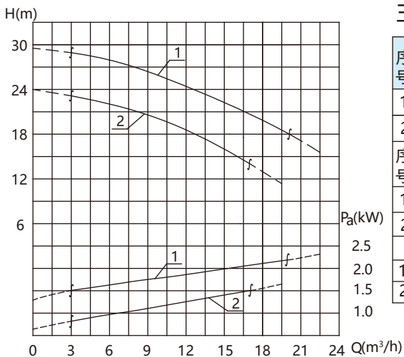
性能曲线图
