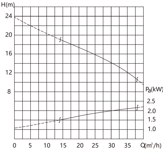
性能曲线图
